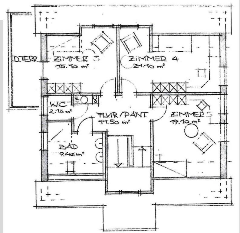
Grundriss Obergeschoss
